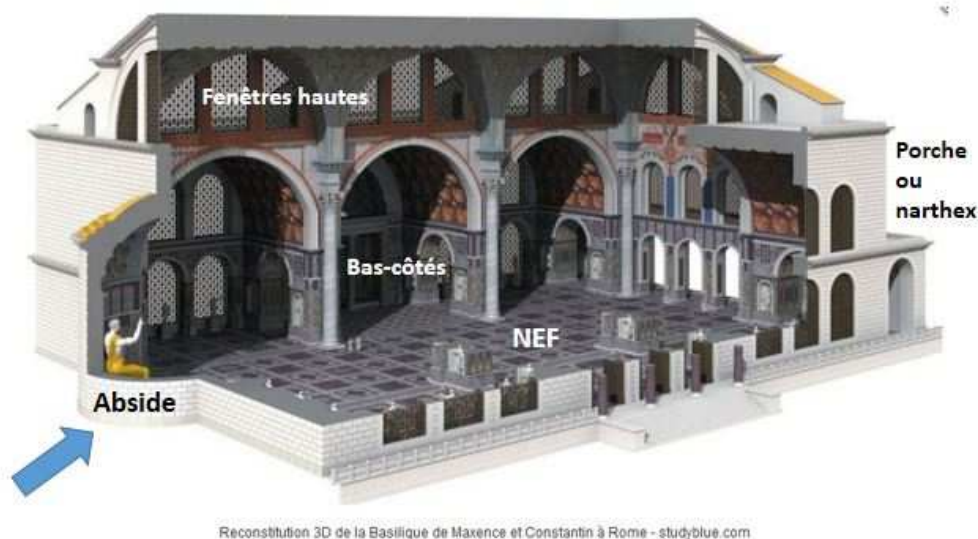
Reconstitution 3D de la Basilique de Maxence et Constantin à Rome - studyblue.com
